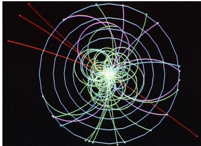
Szimulált Higgs keltés és bomlása 4 müonba (piros vonalak) az LHC-n
